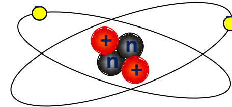
Helium
