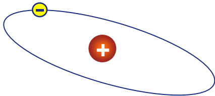
Wasserstoff
