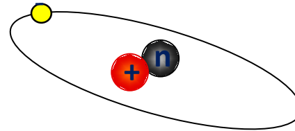
schwererer Wasserstoff
