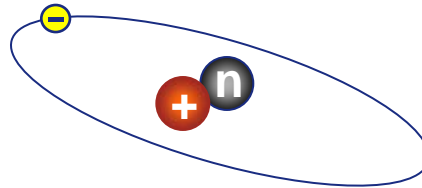
schwerer Wasserstoff
