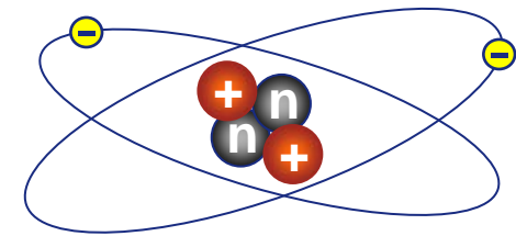
Helium
