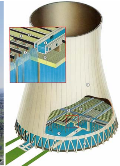
④ Kühlturm
