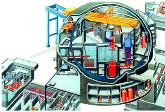
① Reaktorgebäude
