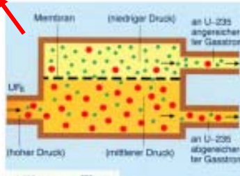
Principe de la diffusion gazeuse
