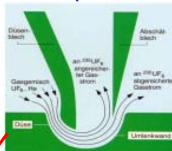
Principe des tuyères de séparation
