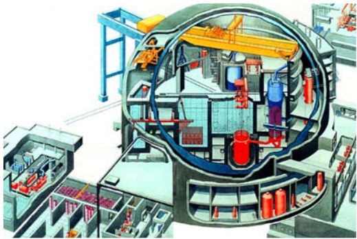
① Bâtiment réacteur
