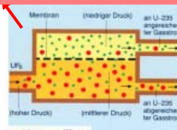
Prinzip Gasdiffusion
