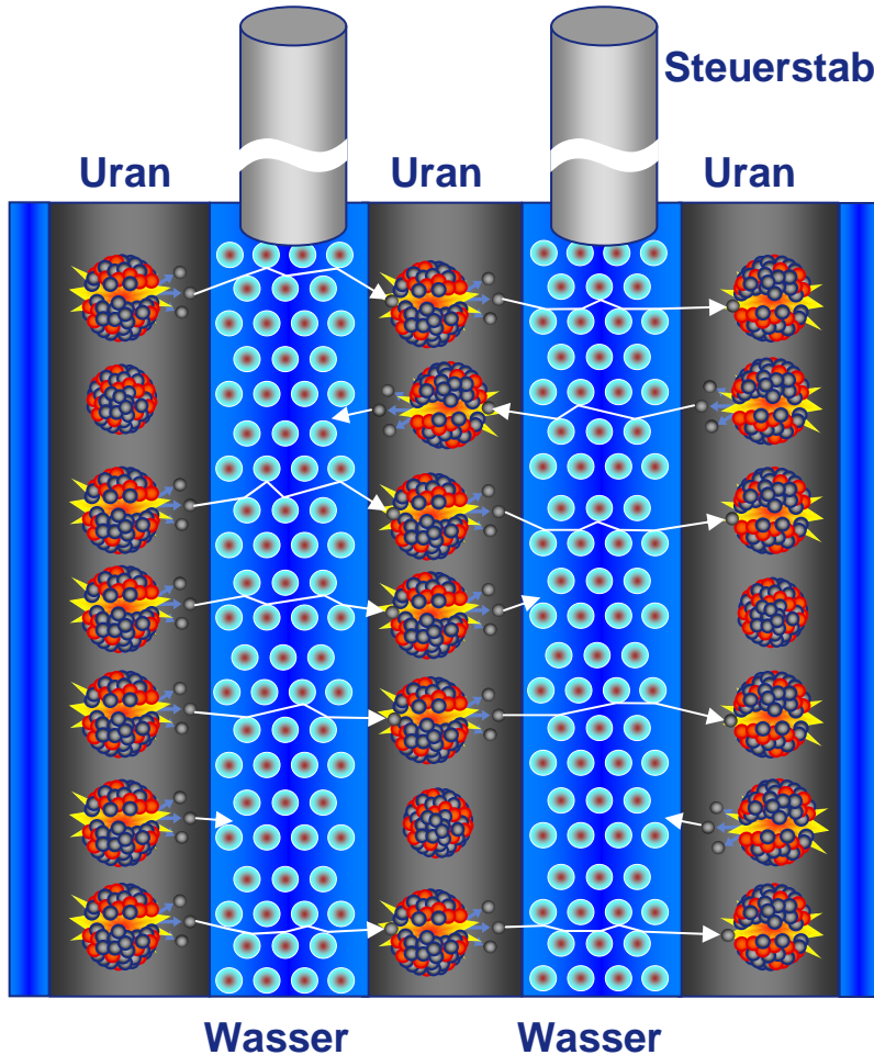
Kettenreaktion ermöglicht
