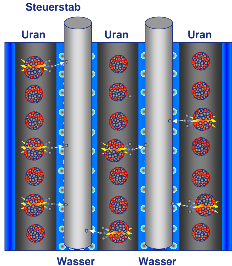
Kettenreaktion unterbrochen
